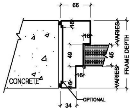
DOUBLE EGRESS DOOR FRAME
