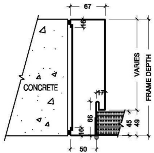
SINGLE RABBETS GROOVE TYPE DOOR FRAME
