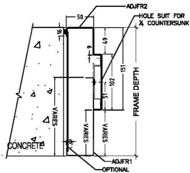
DOUBLE RABBETS ADJUSTABLE DOOR FRAME
